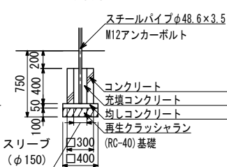
C'2 基礎詳細図
