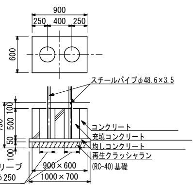
E'基礎詳細図 (スリーブ穴位置や方向に注意する事)
