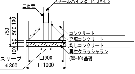
F'基礎詳細図
