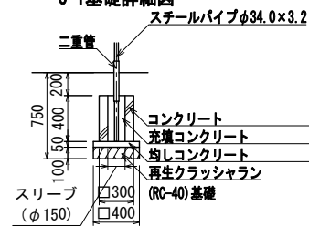
C'1基礎詳細図
