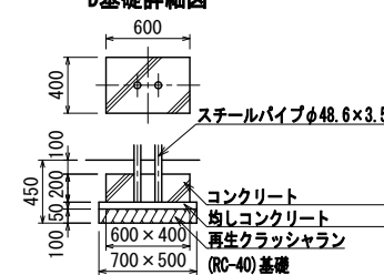
D 基礎詳細図
