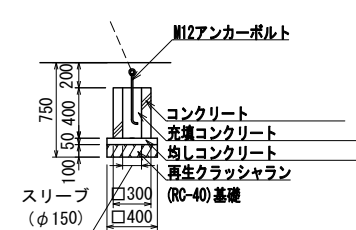
C'2 基礎詳細図
