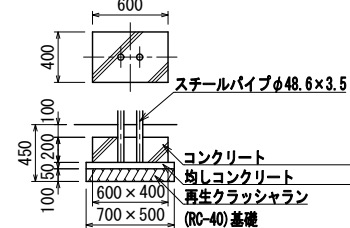
D基礎詳細図
