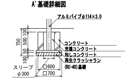
基礎詳細図 S=1:30 (A1) S=1:60 (A3)
