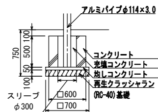
A' 基礎詳細図
