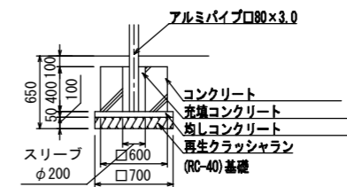
E' 基礎詳細図
