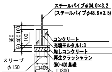
B' 基礎詳細図
