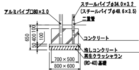
D' 基礎詳細図
