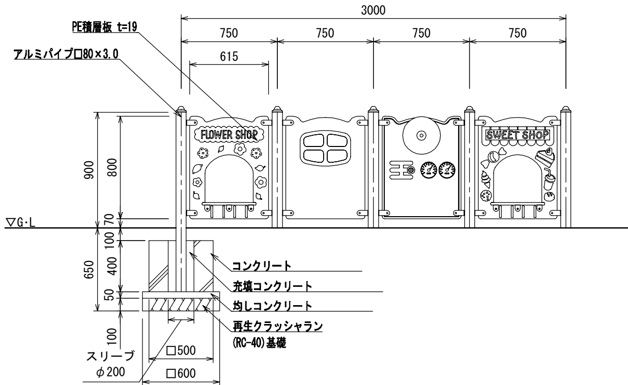
展開図
