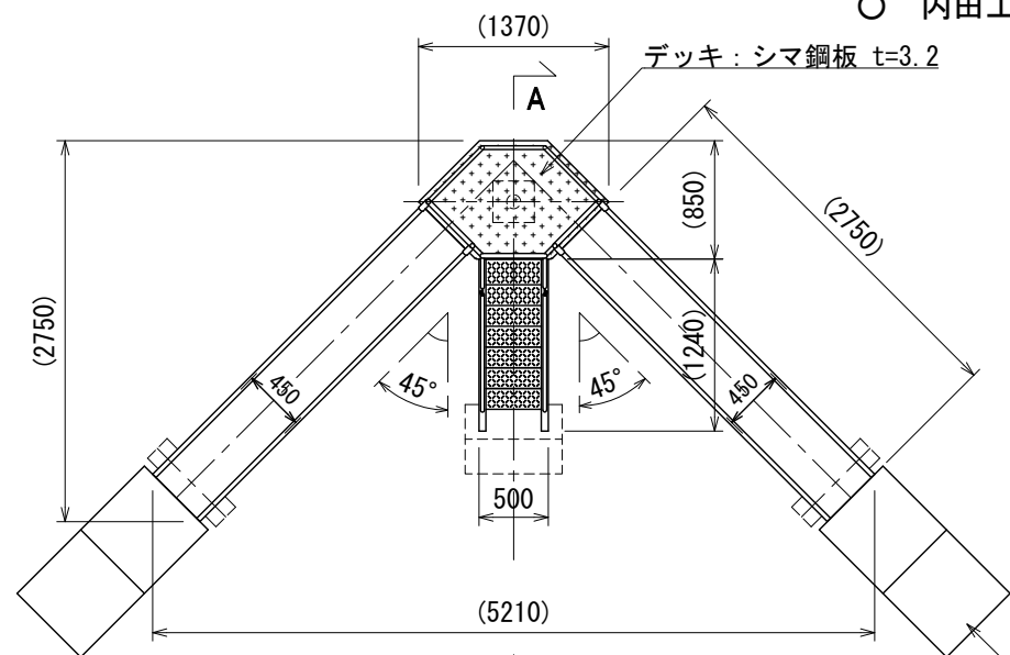
平面図
