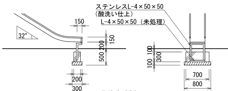
滑降部詳細図
