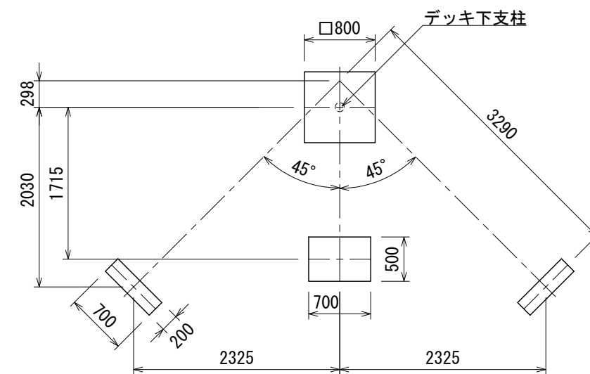
基礎伏図
