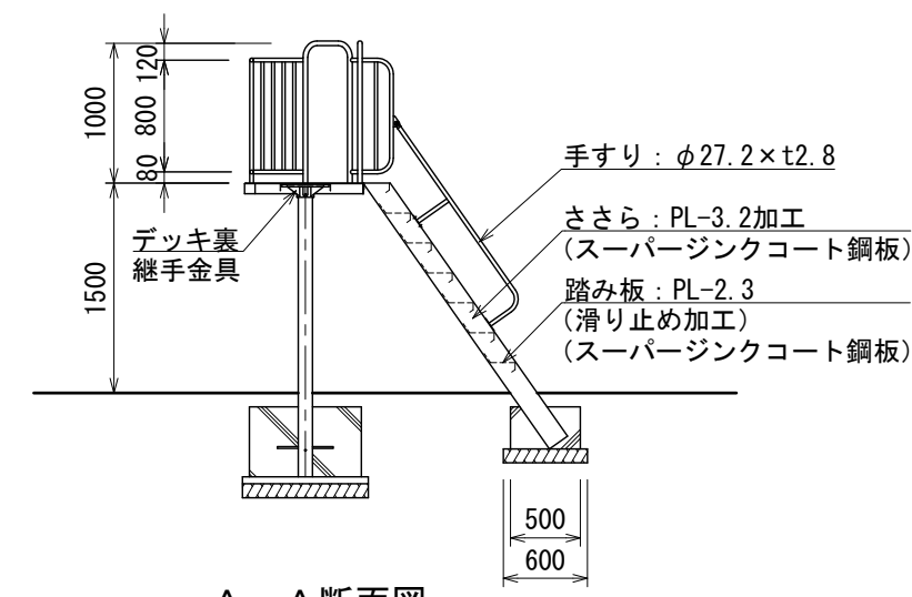
A-A断面図
