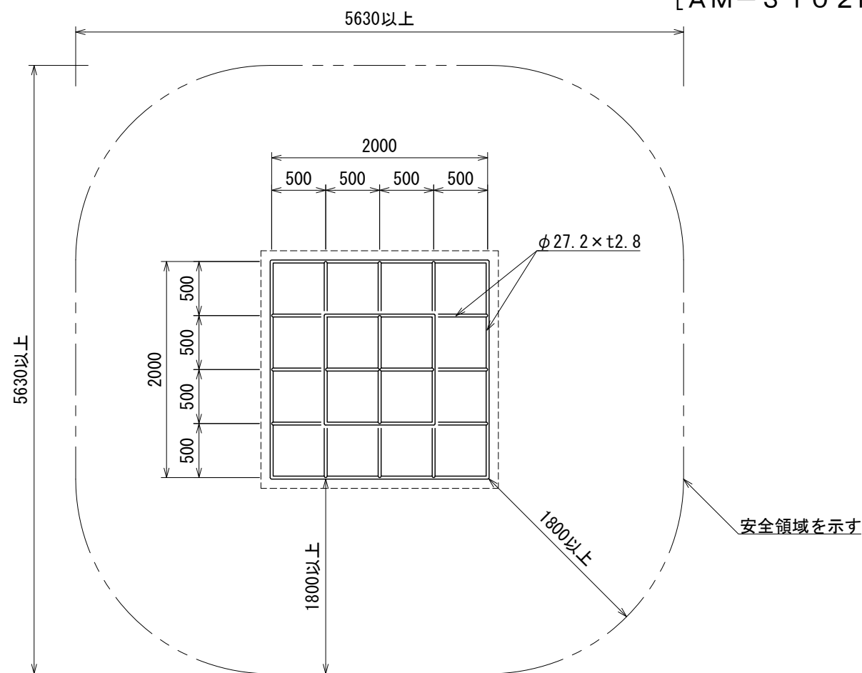
平面図
