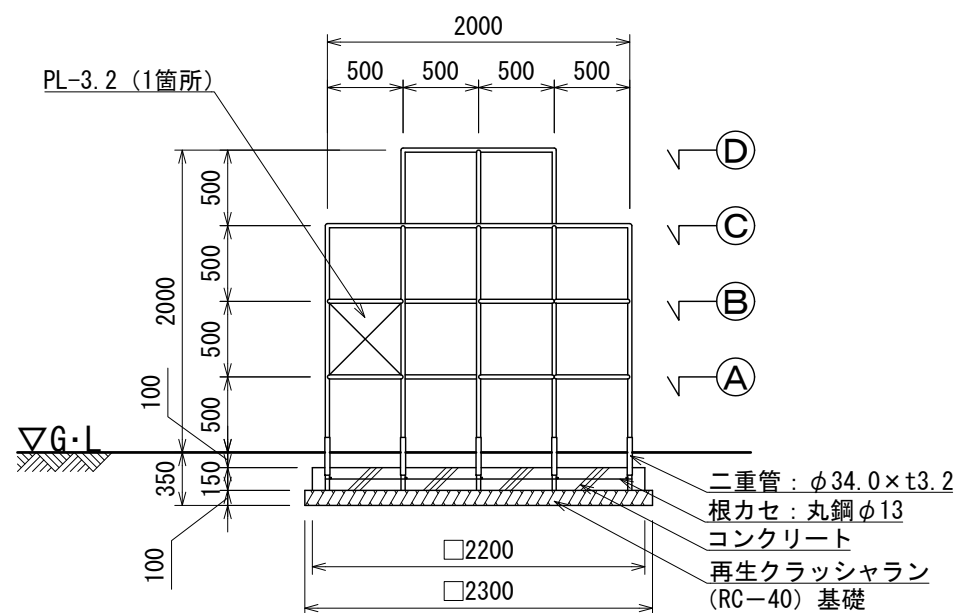
立面図
