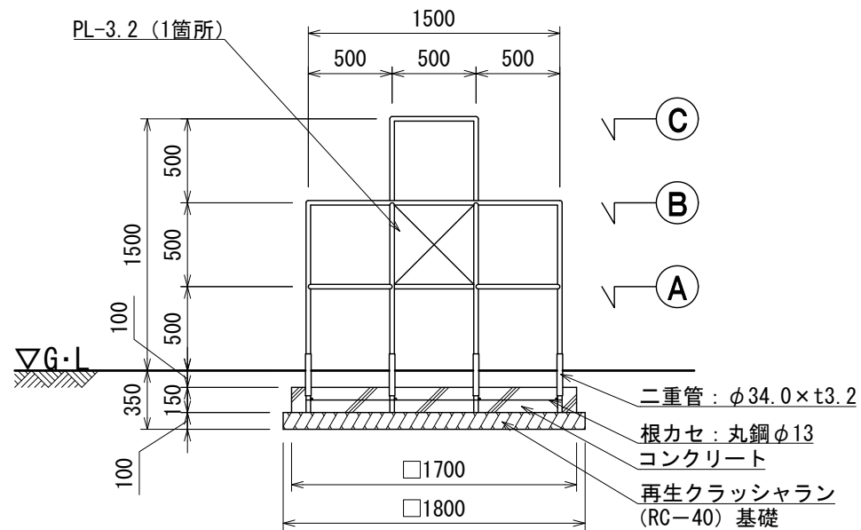
立面図
