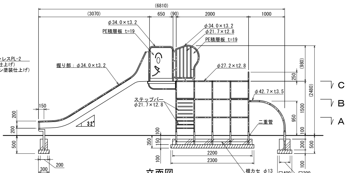
立面図
