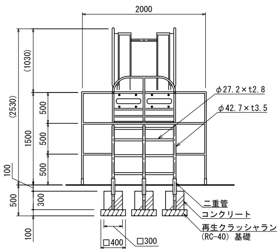
背面図
