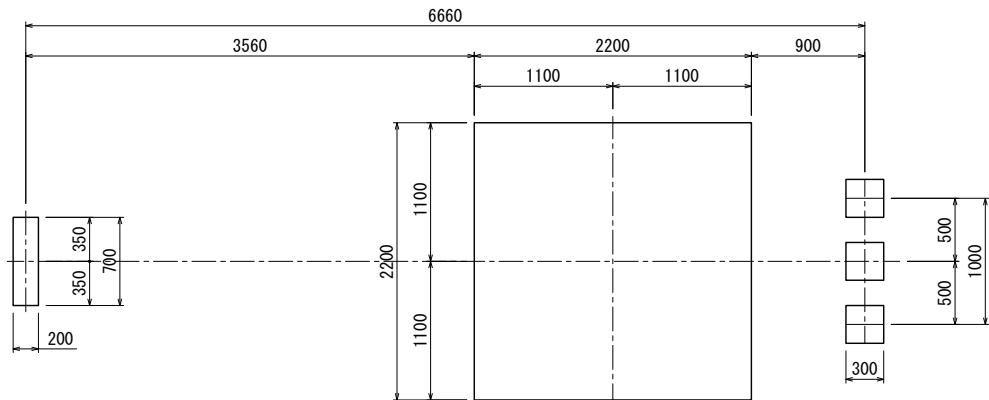
基礎伏図
