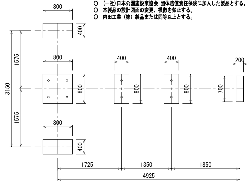
基礎伏図
