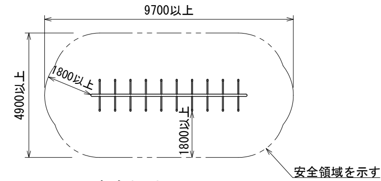
安全領域図 S=1:150
