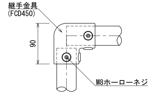
継手金具詳細 S=1:5
