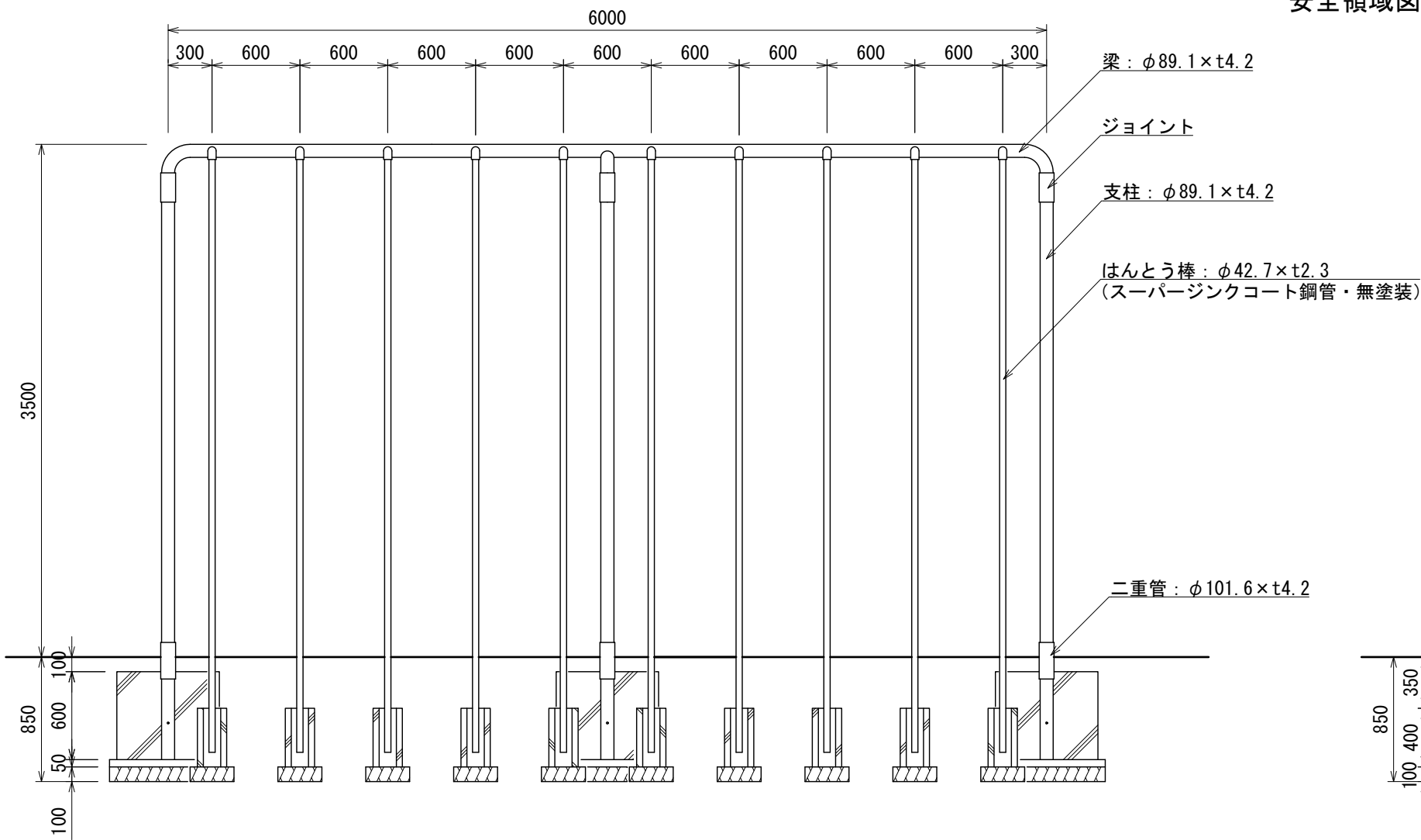
安全領域図 S=1:150
