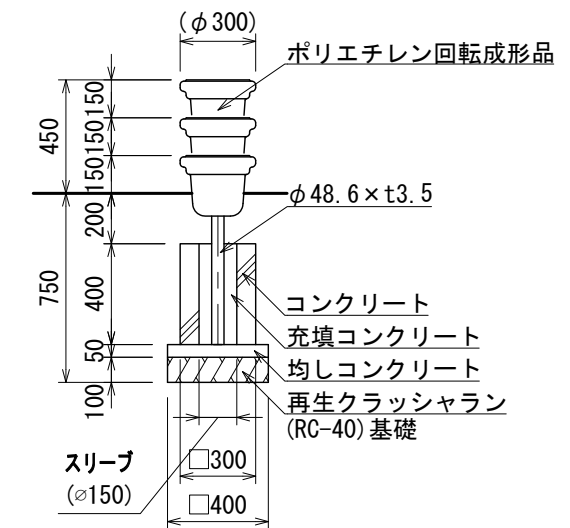
基礎詳細図 S=1:30 (A3)
