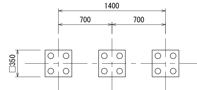
基礎伏図
