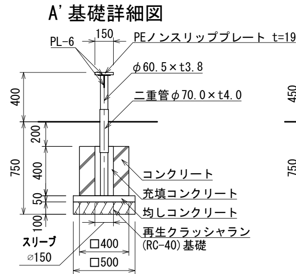
基礎詳細図 S=1:30 (A3)
