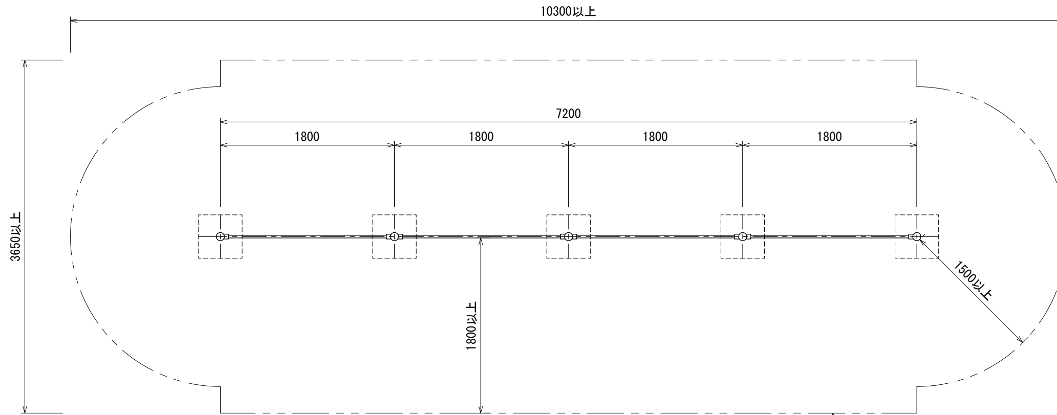
平面図
