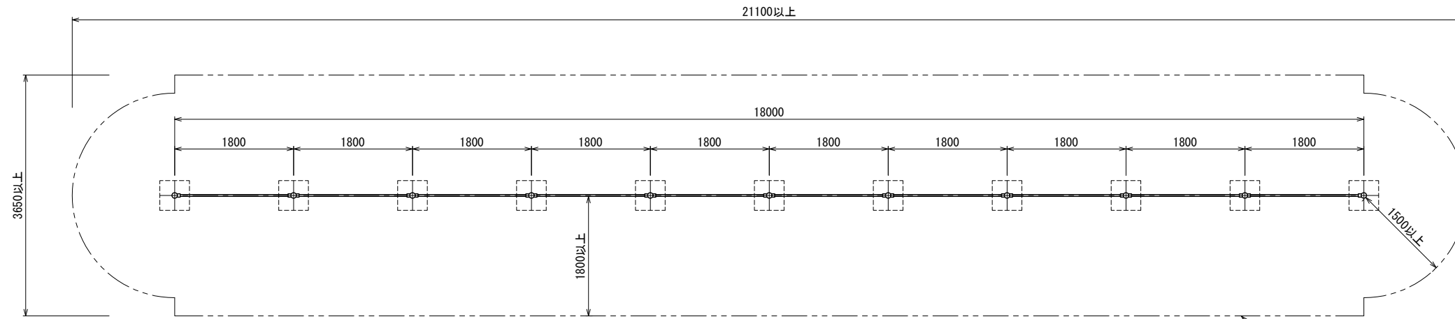
平面図
