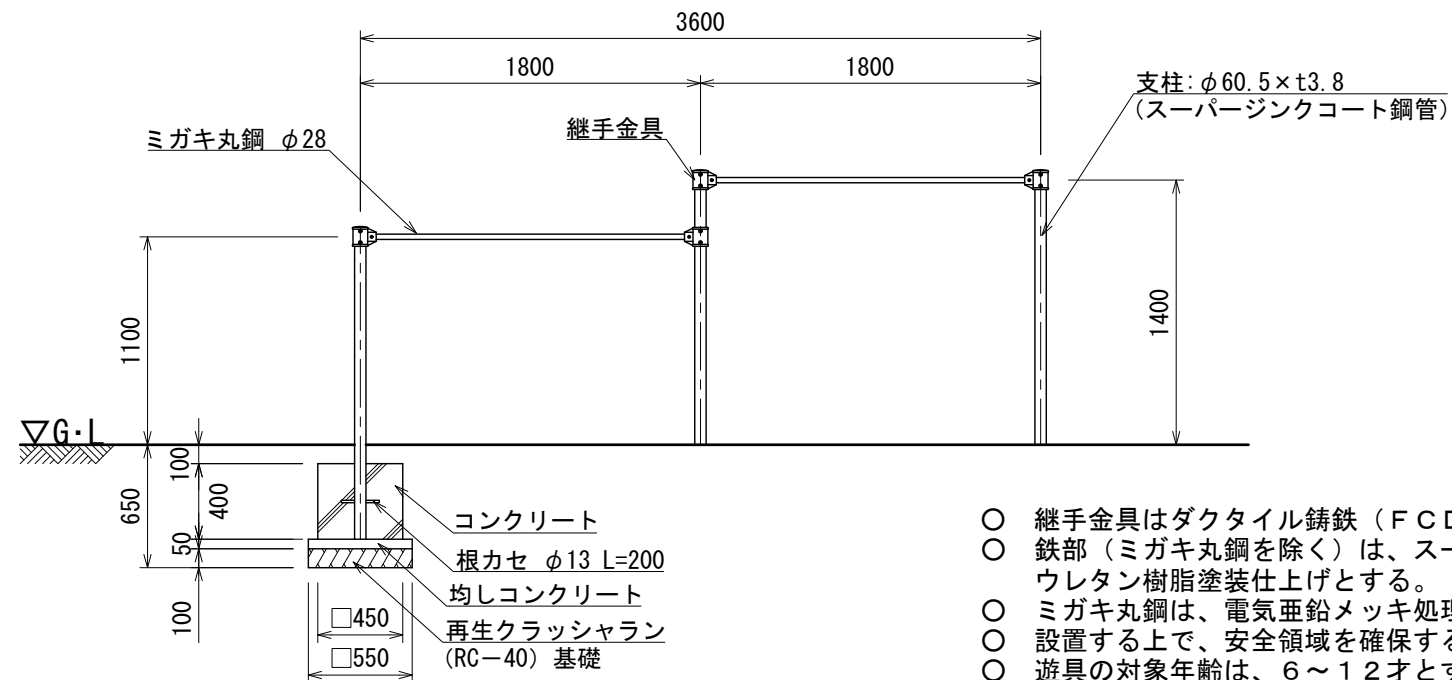
立面図
