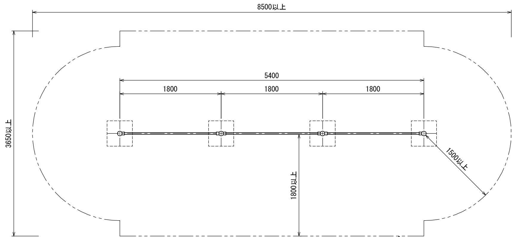
平面図
