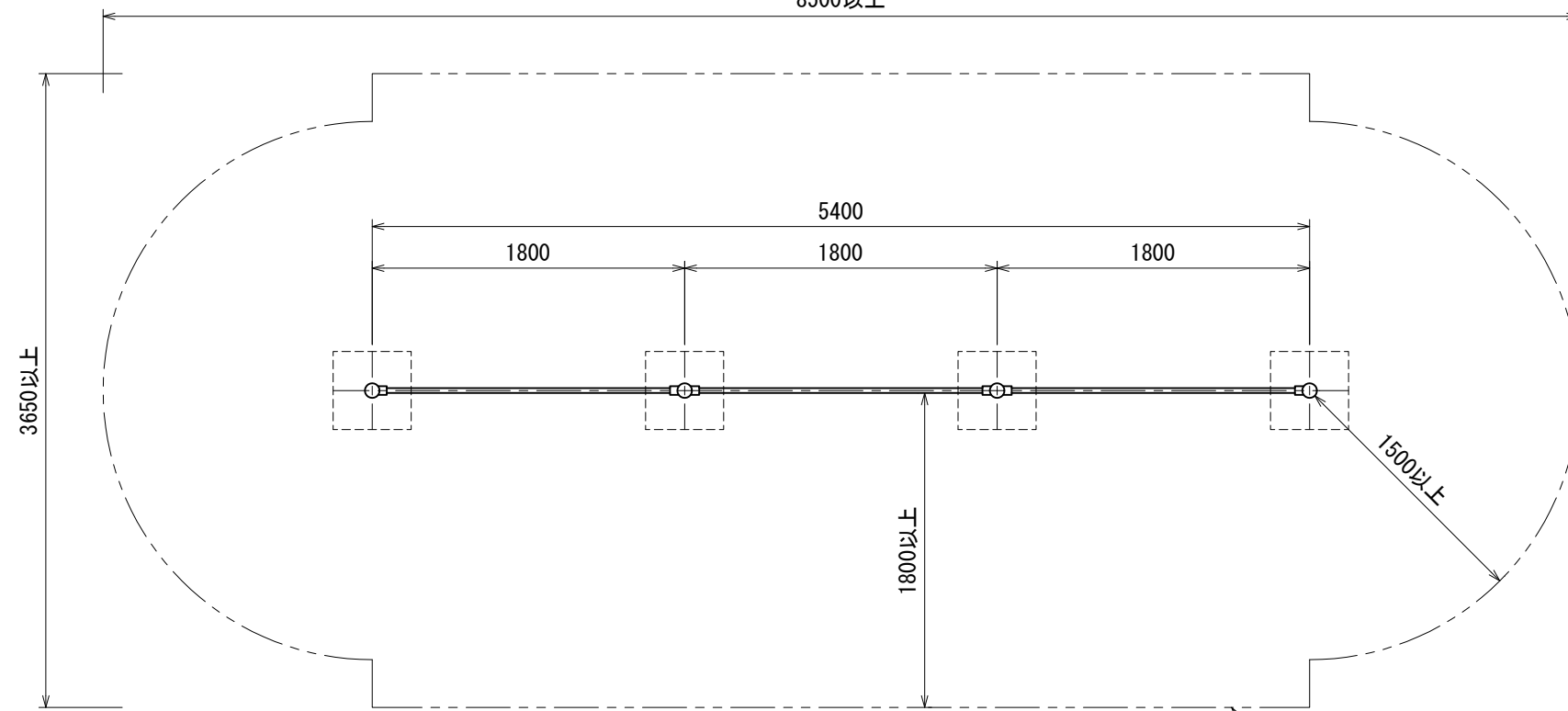
平面図
