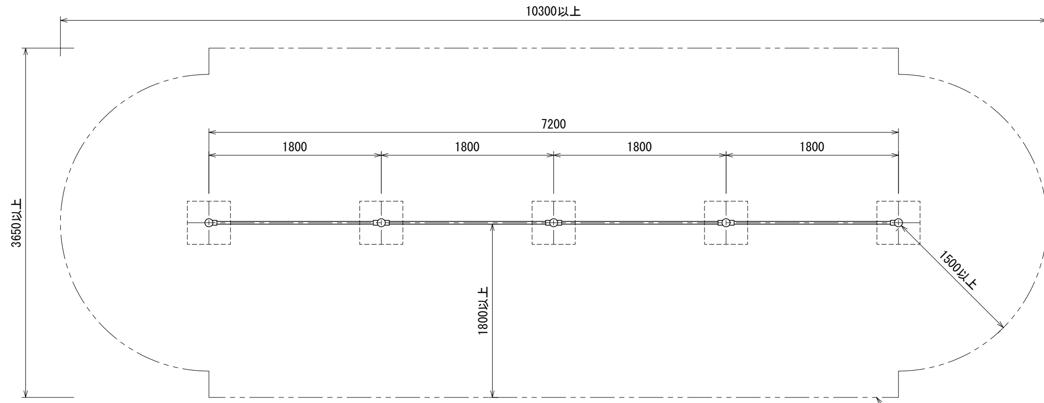
平面図
