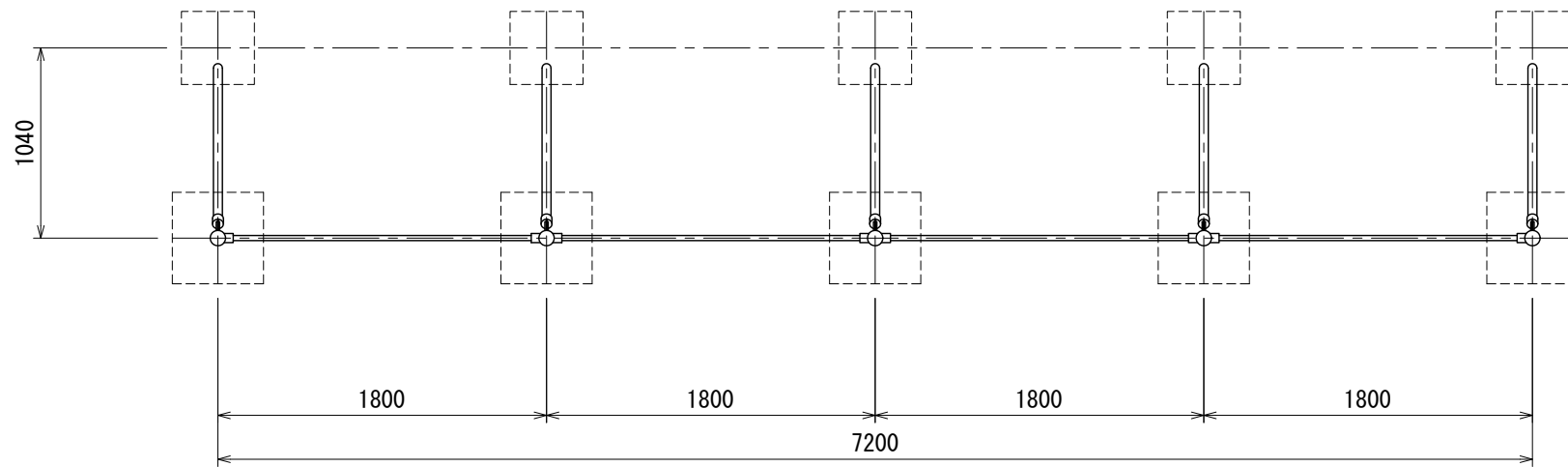
平面図
