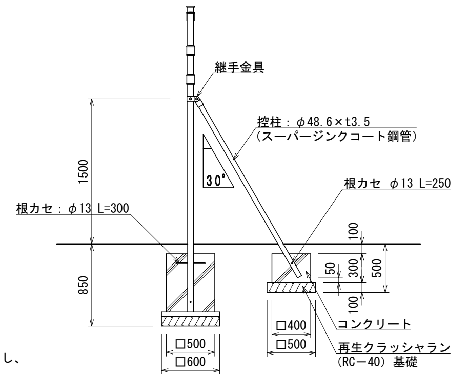
側面図
