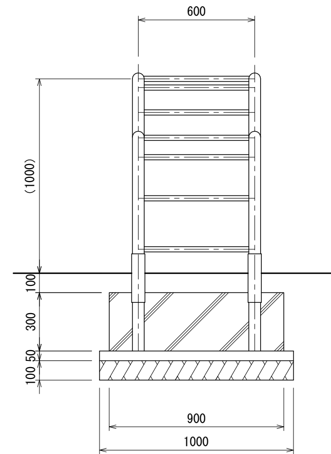
安全領域図 S=1:100
