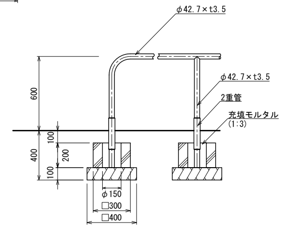
C基礎
