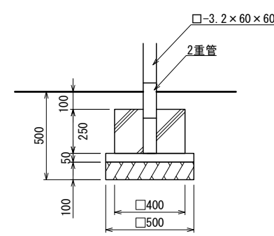
B基礎
