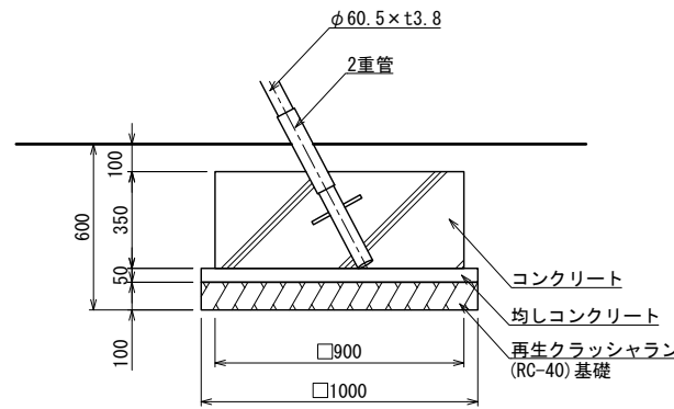
A基礎
