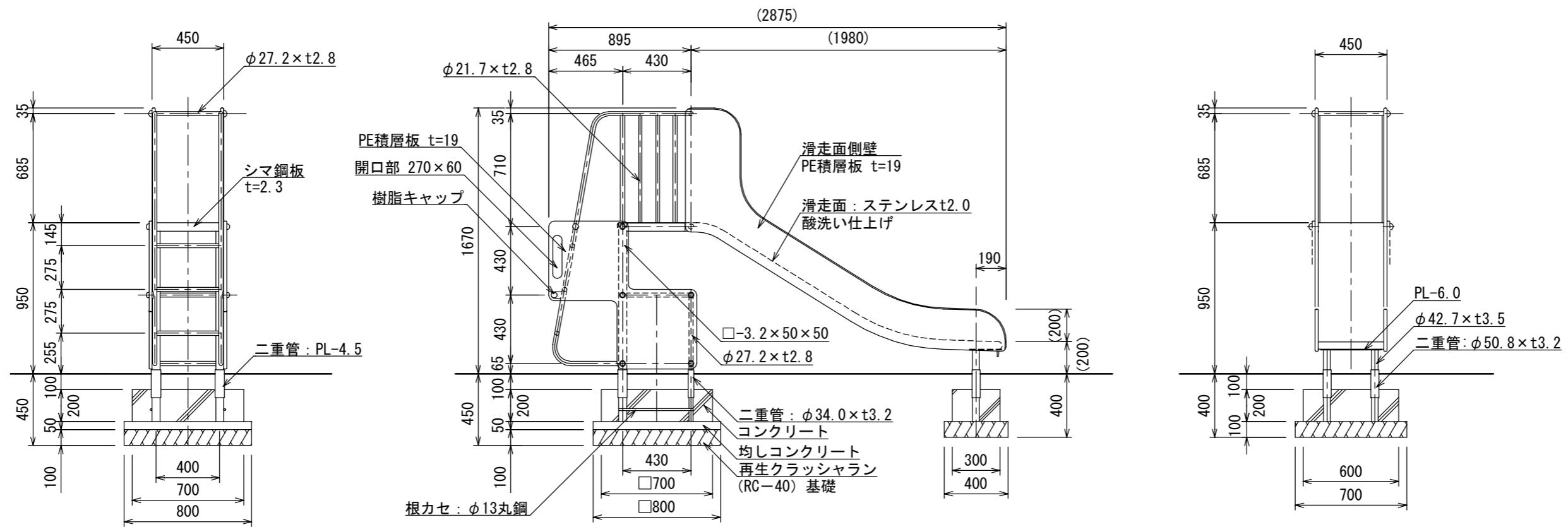
安全領域図 S=1:100
