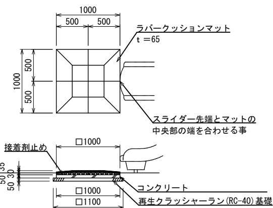
ラバークッションマット詳細図 S=1:30 (A3 S=1:60)
