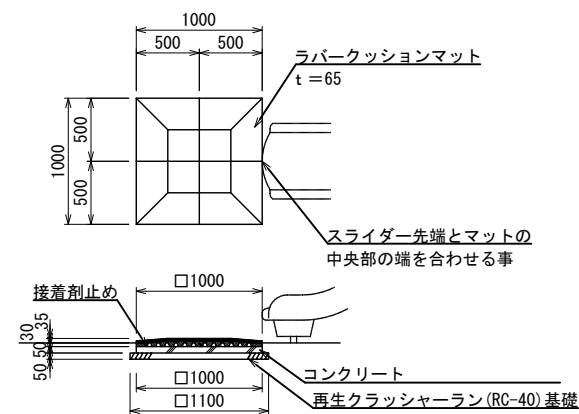
オプション ラバークッションマット詳細図 [AO-9112]
