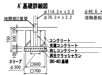
基礎詳細図 S=1:30 (A3 S=1:60)
