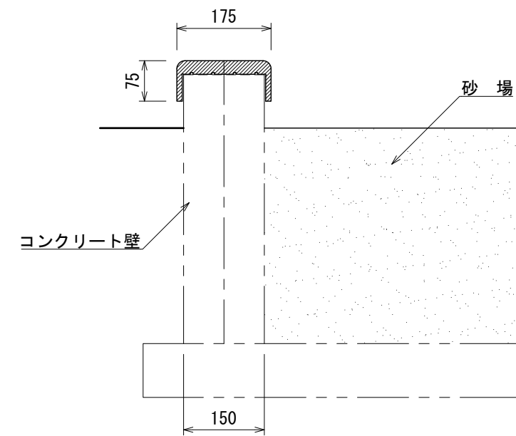
標準断面図
