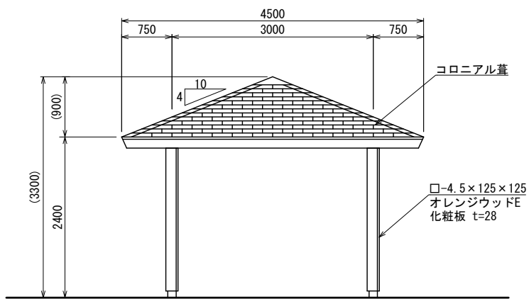
立面図
