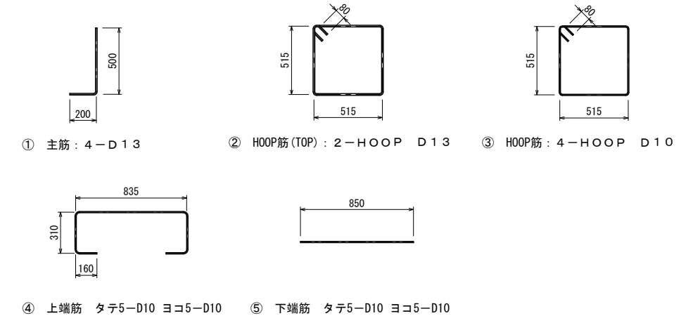
鉄筋図 S=1:20 (A3 S=1:40)
