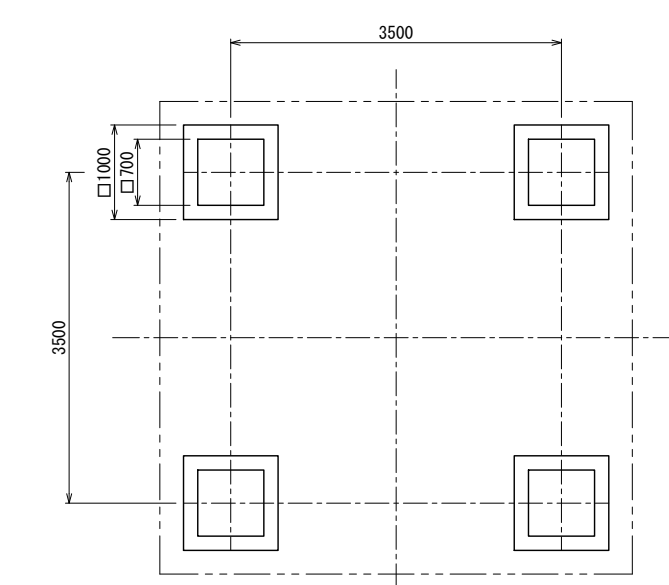
基礎伏図
