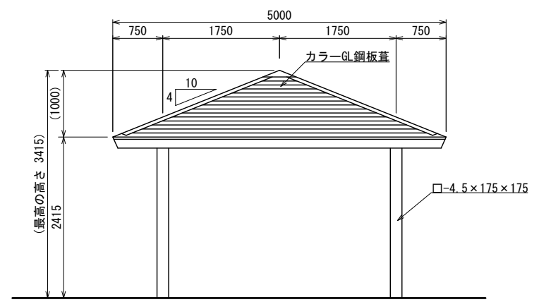
立面図
