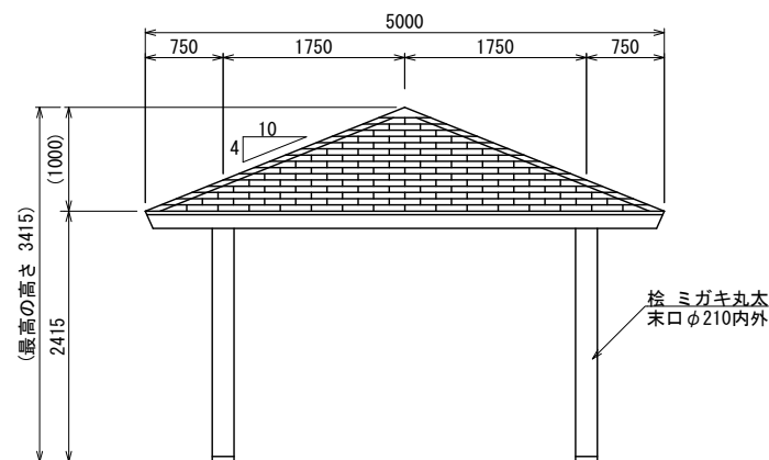
立面図
