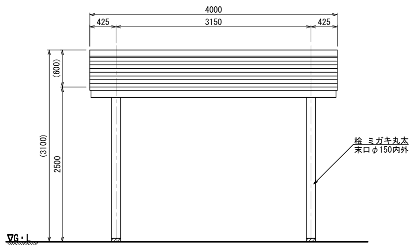
立面図
