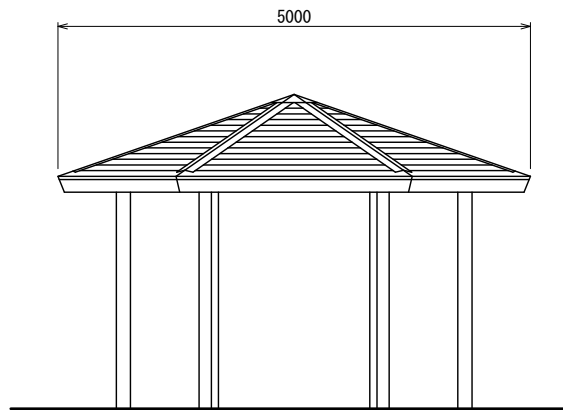
側面図
