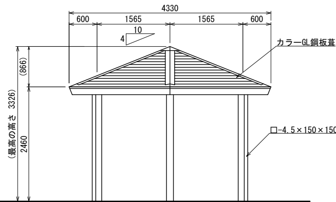
立面図
