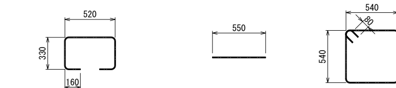
① 上端筋 タテ・ヨコ共 2-D10 ② 下端筋 タテ・ヨコ共 2-D10 ③ HOOP 2-D10
