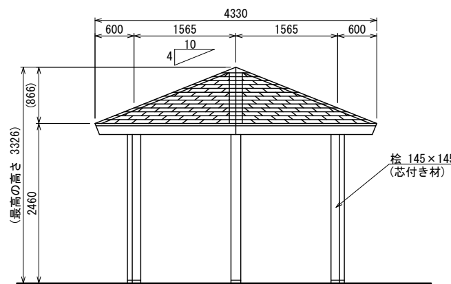
立面図
