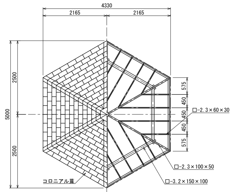
平面図
