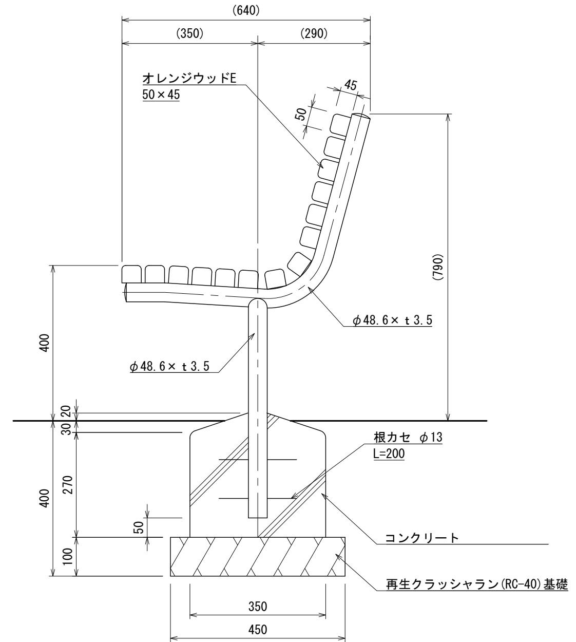
[座部断面図(2層構造)]
