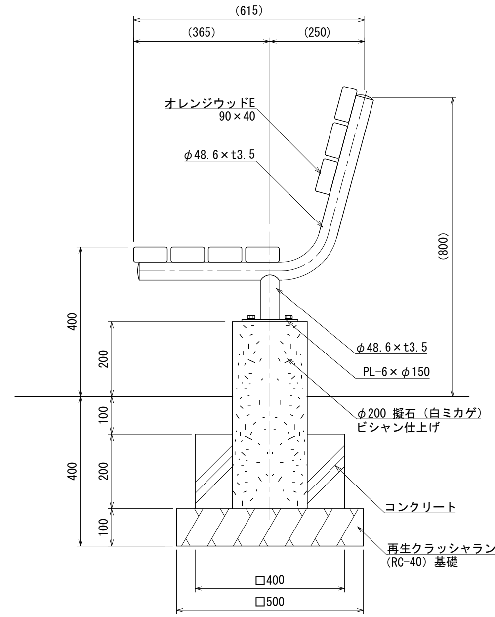
[座部断面図(2層構造)]
