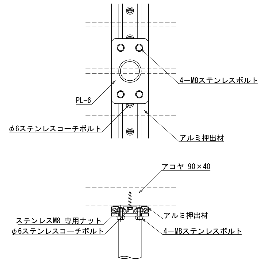
支柱取付詳細図 S=1:5
