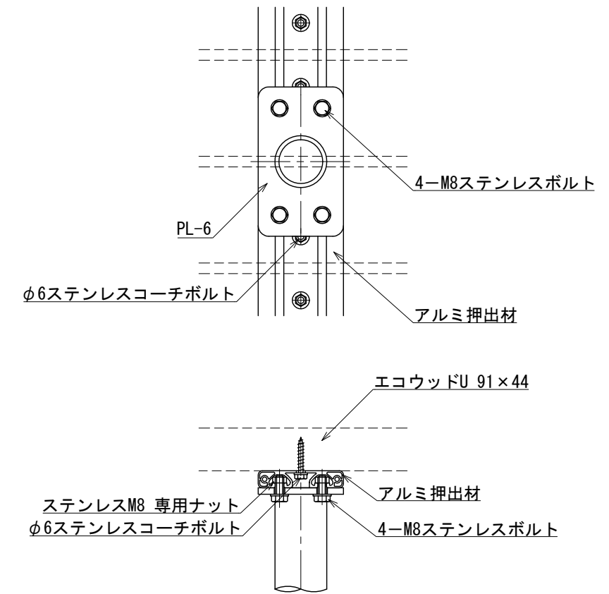
支柱取付詳細図 S=1:5
