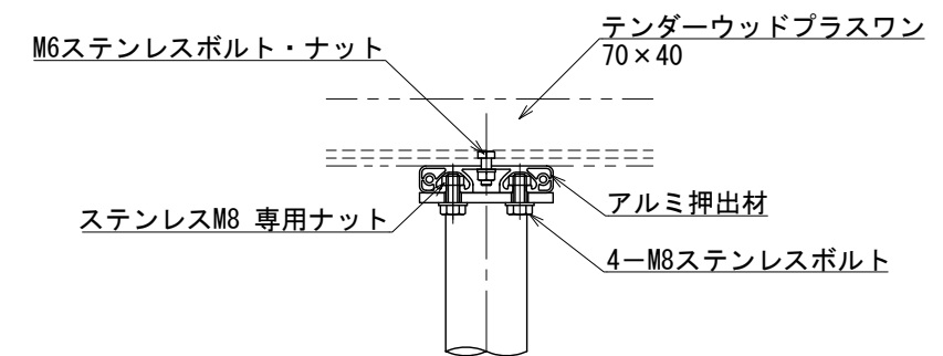
支柱取付詳細図 S=1:5
