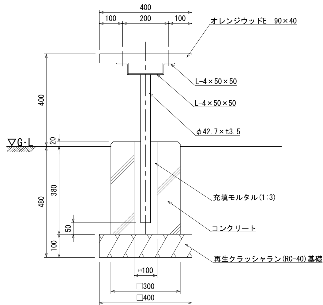
断面詳細図 S=1:10
