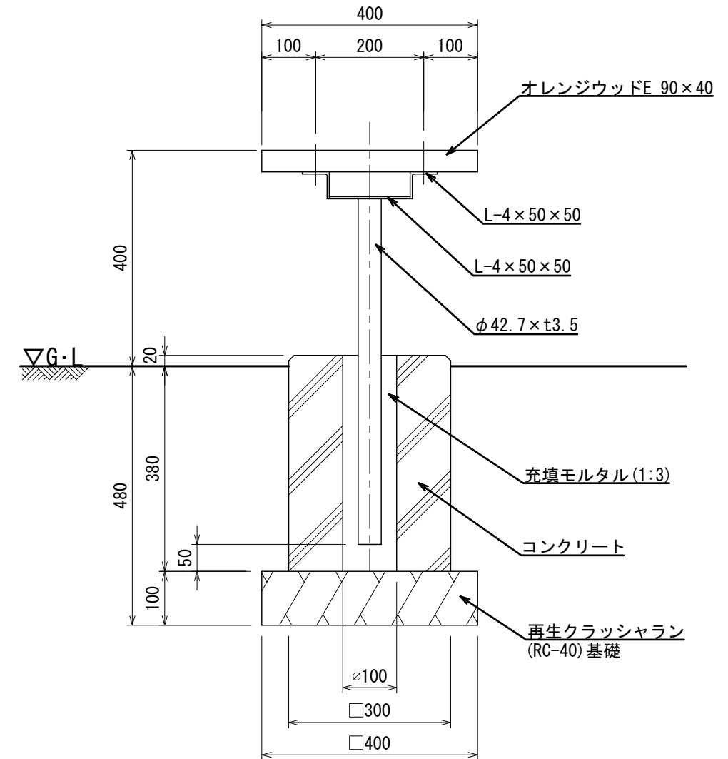
断面詳細図 S=1:10
