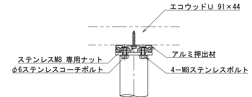
支柱取付部詳細図 S=1:5
