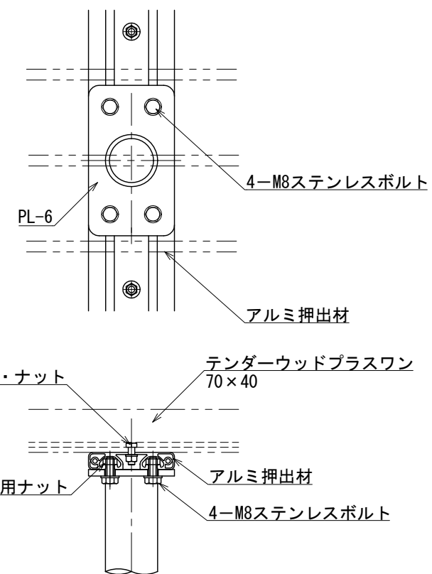
支柱取付部詳細図 S=1:5
