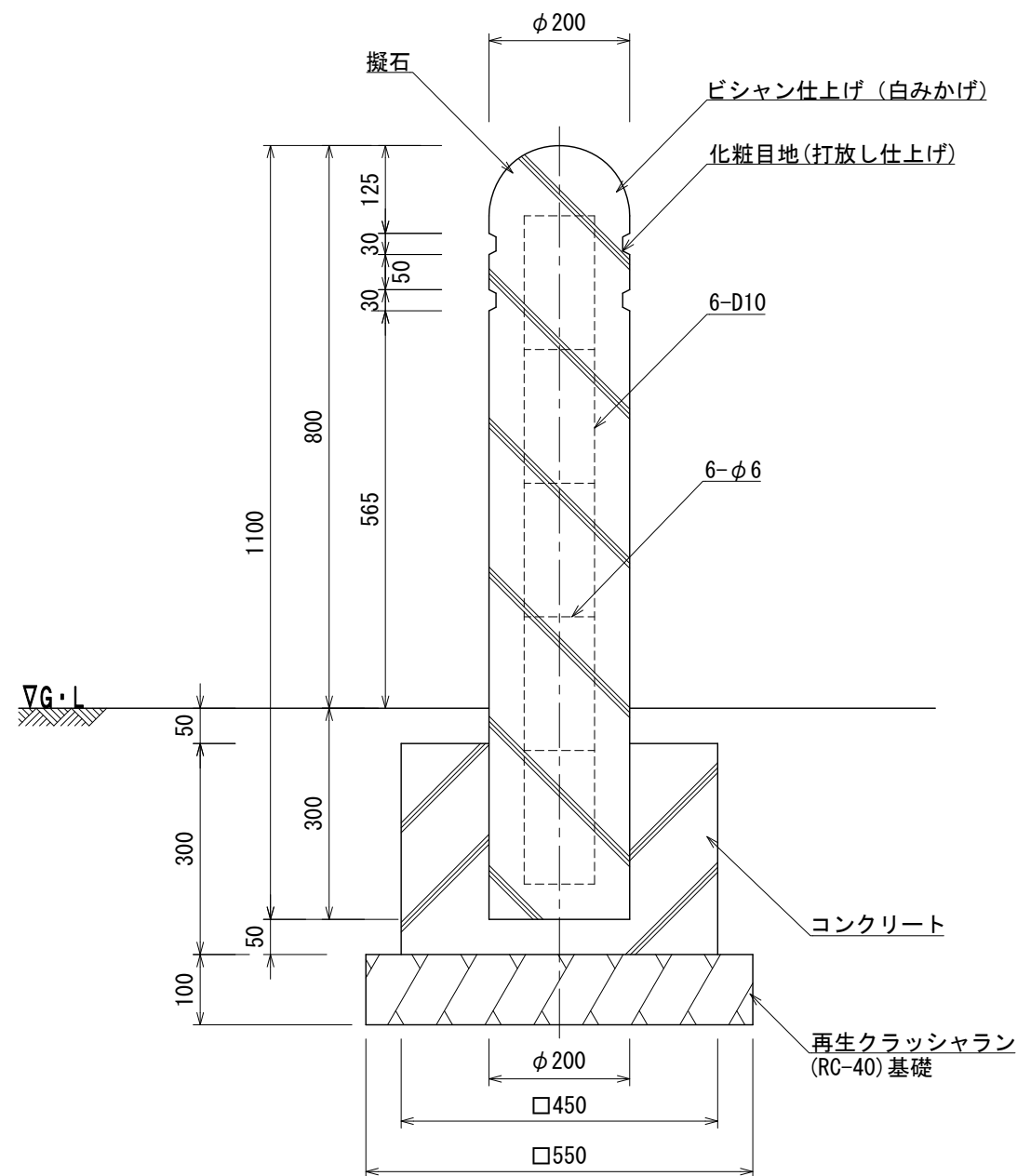
断面図
