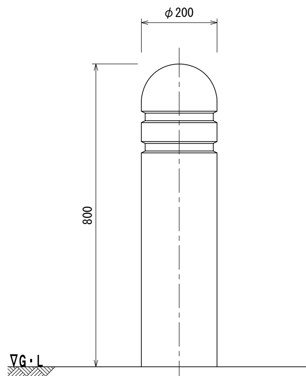
立面図
