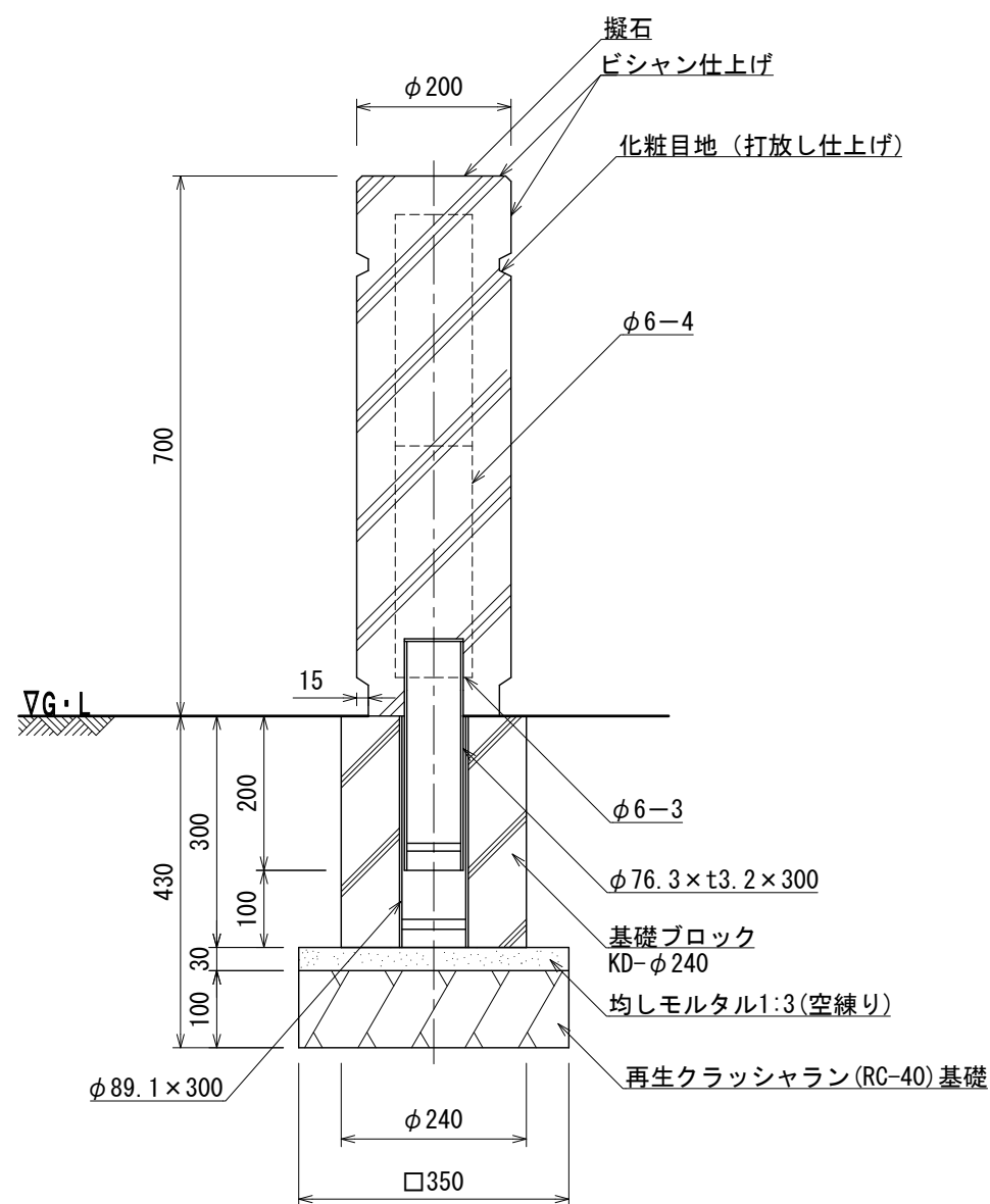
断面図
