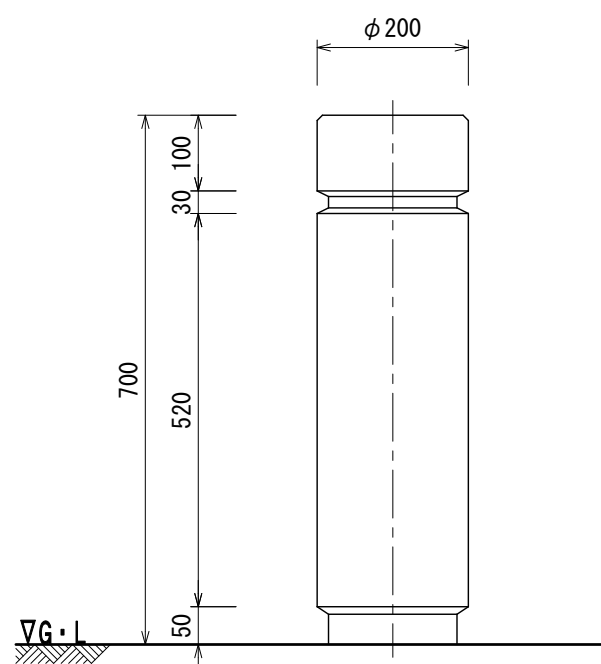
立面図
