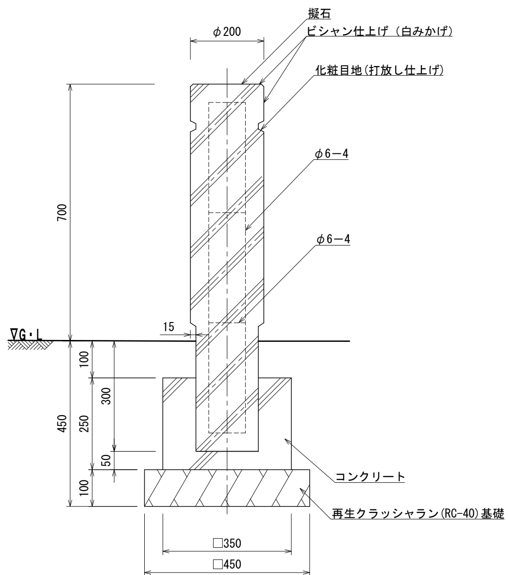
断面図
