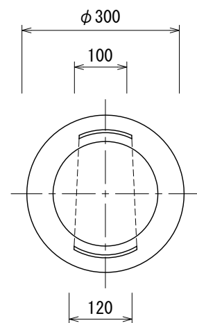
平面図
