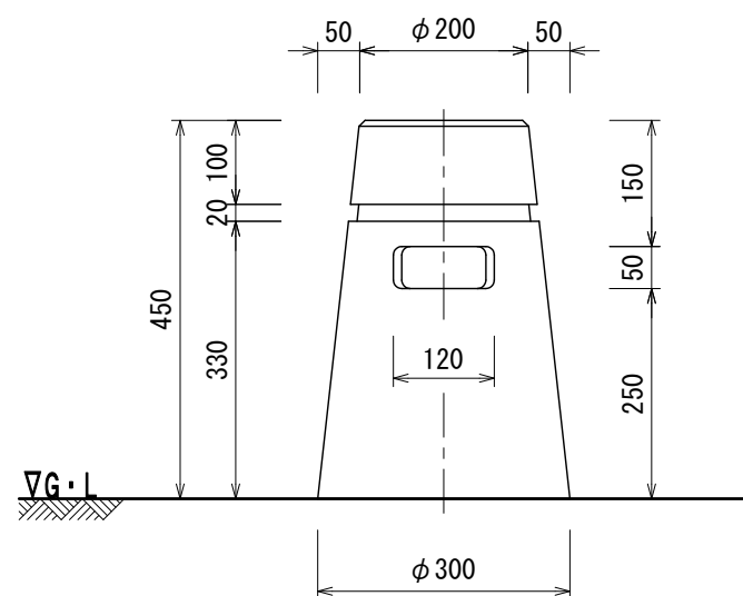
立面図
